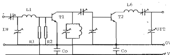
FIGUUR 2 HET WISSELSTROOMSCHEMA
