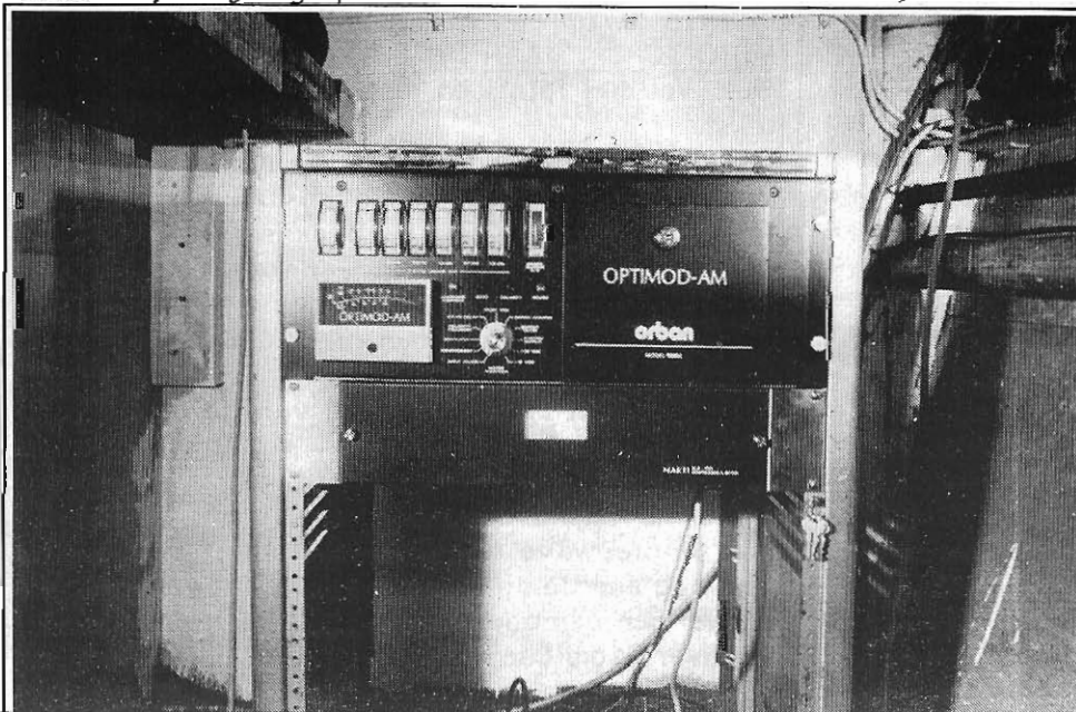
De Orban Optimod en Marti limiter/kompressor
