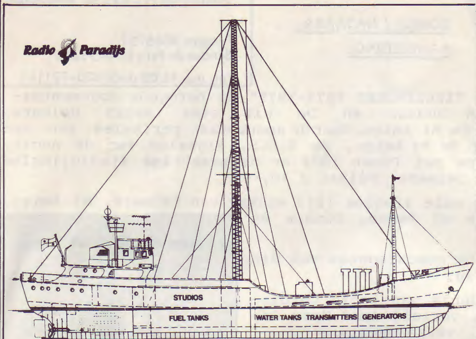
Tekening van de opbouw en indeling van het zendschip van Radio Paradijs, de "Magda Maria" van Elke Kampen. (Medewerkster "Radio News").
