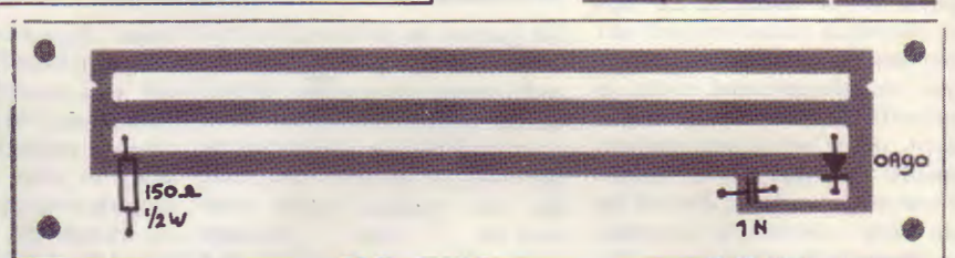
PRINTLAYOUT (koperzijde)
