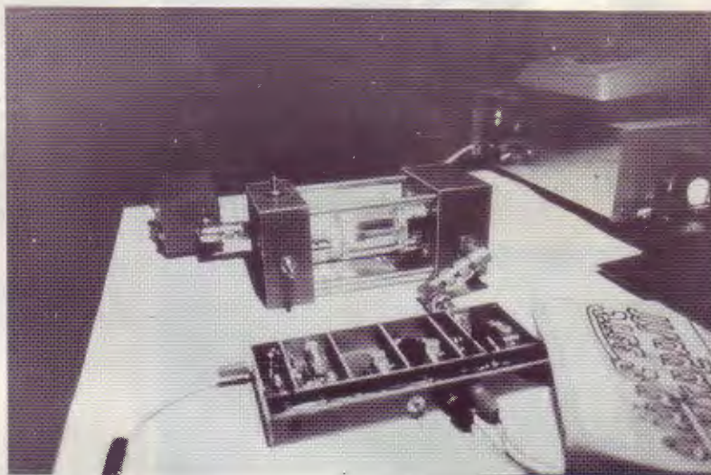
"De zender" van een QSO-station uit Delft: een viertraps-transistorzender (MRF237) en de eindbuis QQE 06/40 met een vermogen van ca. 75 Watt.
