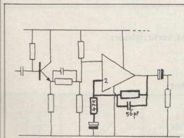
Verbeterd schema Multiplex FRM 4-'82
