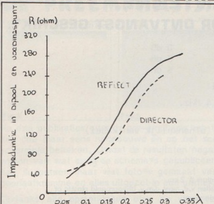
FIG. 1. AFSTAND VAN DIRECTOR EN REFLECTOR t.o.v. het hoofdelement
