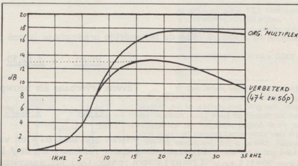
Verbeterd schema Multiplex FRM 4-'82
