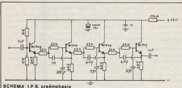
SCHEMA I.P.S. preëmphasis
