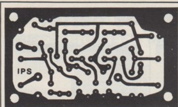
Print lay-out
