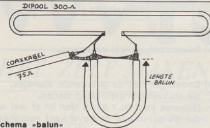
Schema »balun«
