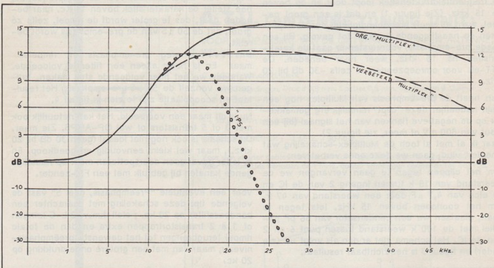
SCHEMA I.P.S. preëmphasis
