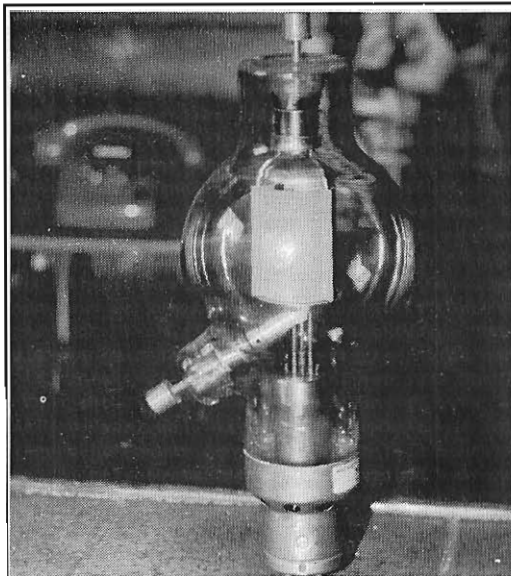
Zendbuis TL 4685
