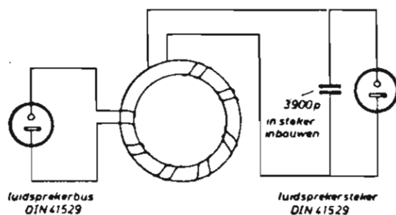
afb. 16 Ontstoringadaptor voor de luidsprekeraansluiting Ferrocard R.K.
