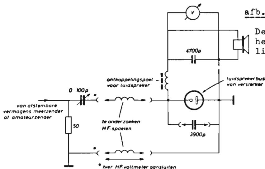
afb. 16 Ontstoringadaptor voor de luidsprekeraansluiting Ferrocard R.K.
