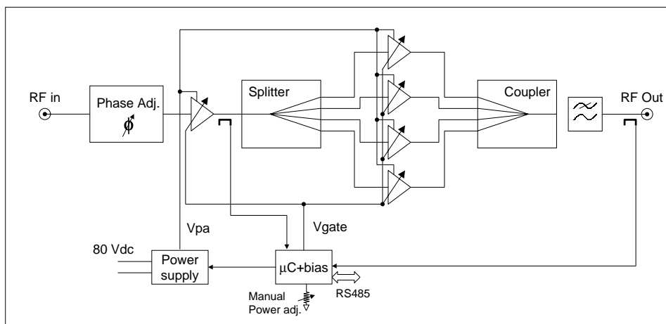
Figura 7-21 Scheda a blocchi di un modulo amplificatore RF
