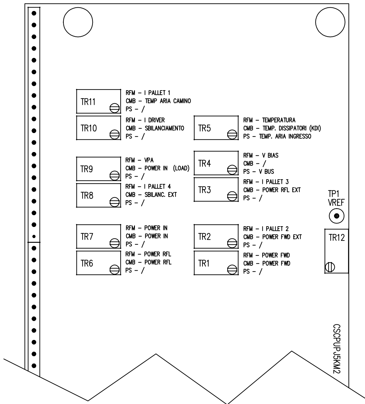
Figura 8-1 Trimmers scheda microcontrollore
