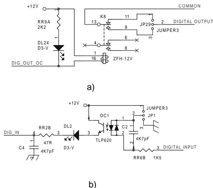
Figura 7-14 Digital I/O
