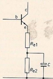
Afb. 10. Tegenkoppeling met „opgedeelde” emitterweerstand.
