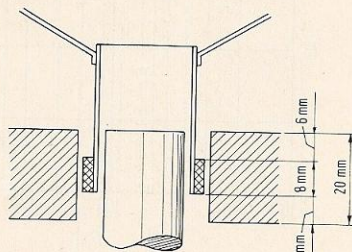
Afb. 2: Een korte spoel in een lange luchtpleet waarborgt een constant magnetisch veld in de spoel.
