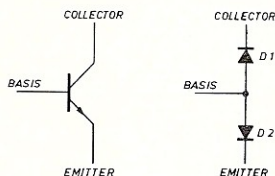
Afb. 4b. NPN-transistor
