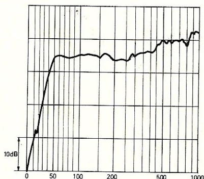
Frequentiearakteristiek van de „Bombardon” (AD 1255/W8)
