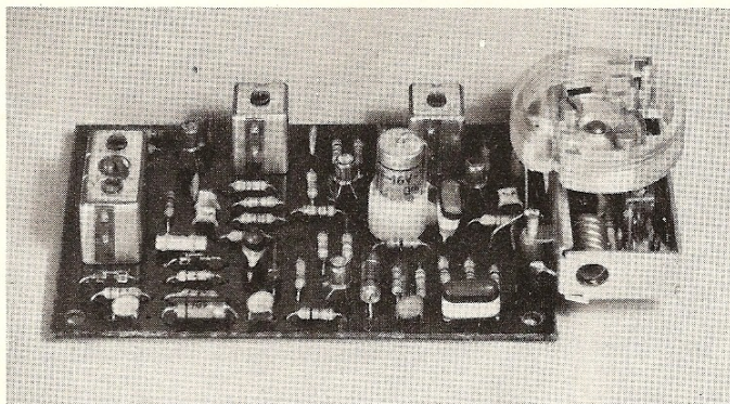
Afb. 2 De gemonteerde FM-afstemeenheid R 6813
