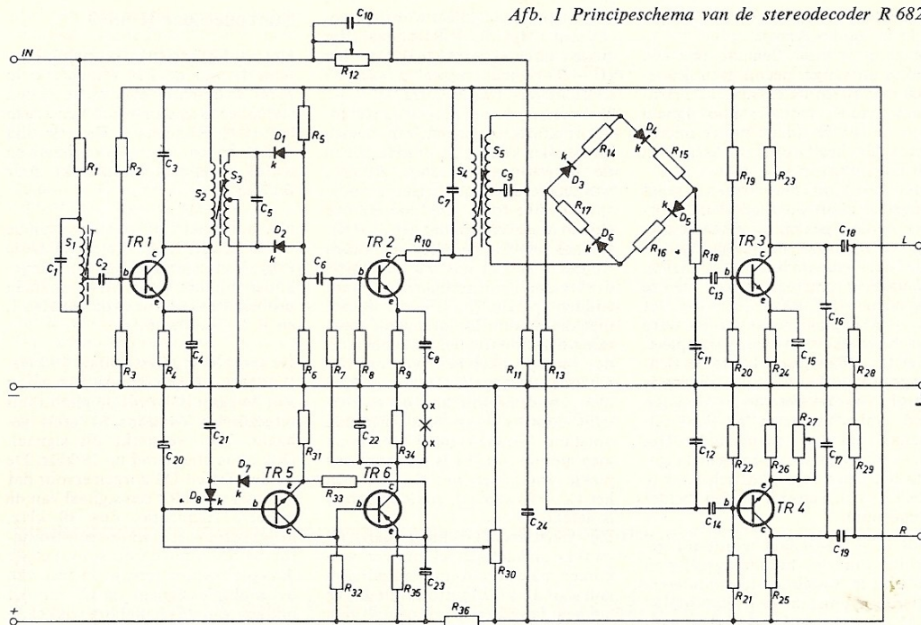
Afb. 1 Principeschema van de stereodecoder R 6823
