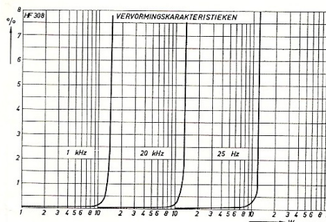
Vervormingskarakteristiek versterker HF 308
