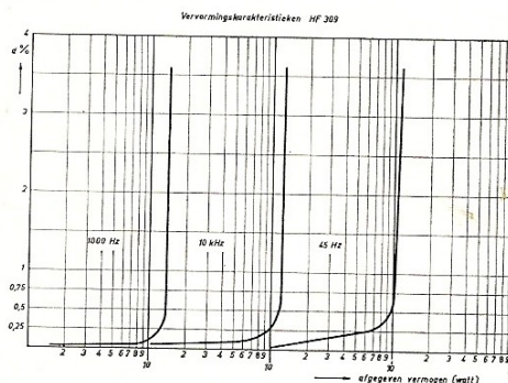
Vervormingskarakteristiek eindversterker HF 309
