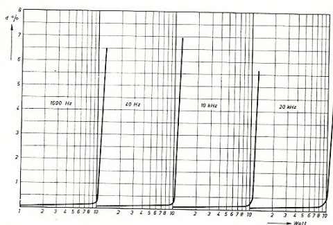
Vervormingskarakteristiek versterker HF 310
